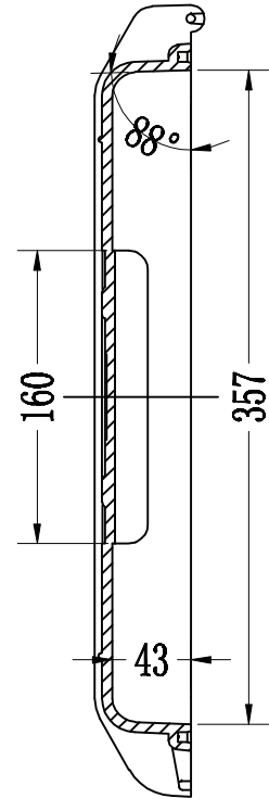
B-B
